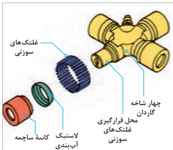
شکل ۳-۵ اجزای ساختمان چهارشاخه گاردان
