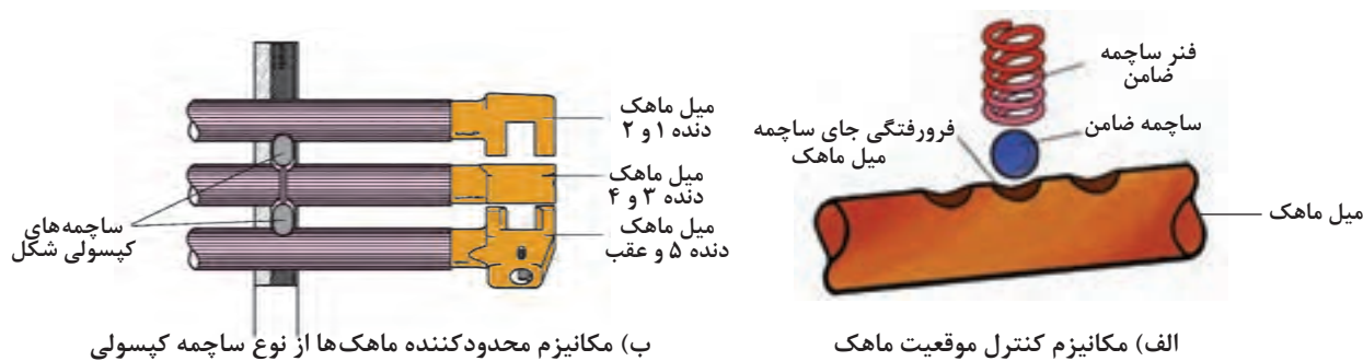
شکل ۱۹-۲- کنترل حرکت ماهک و میل ماهک
