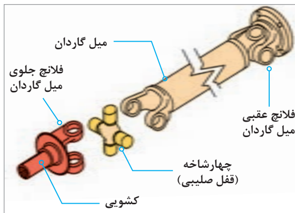
شکل ۳-۴ نحوه اتصال چهارشاخه گاردان به سایر اجزا
