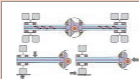
شکل ۱۴-۵ انواع یاتاقان بندی پلوس
